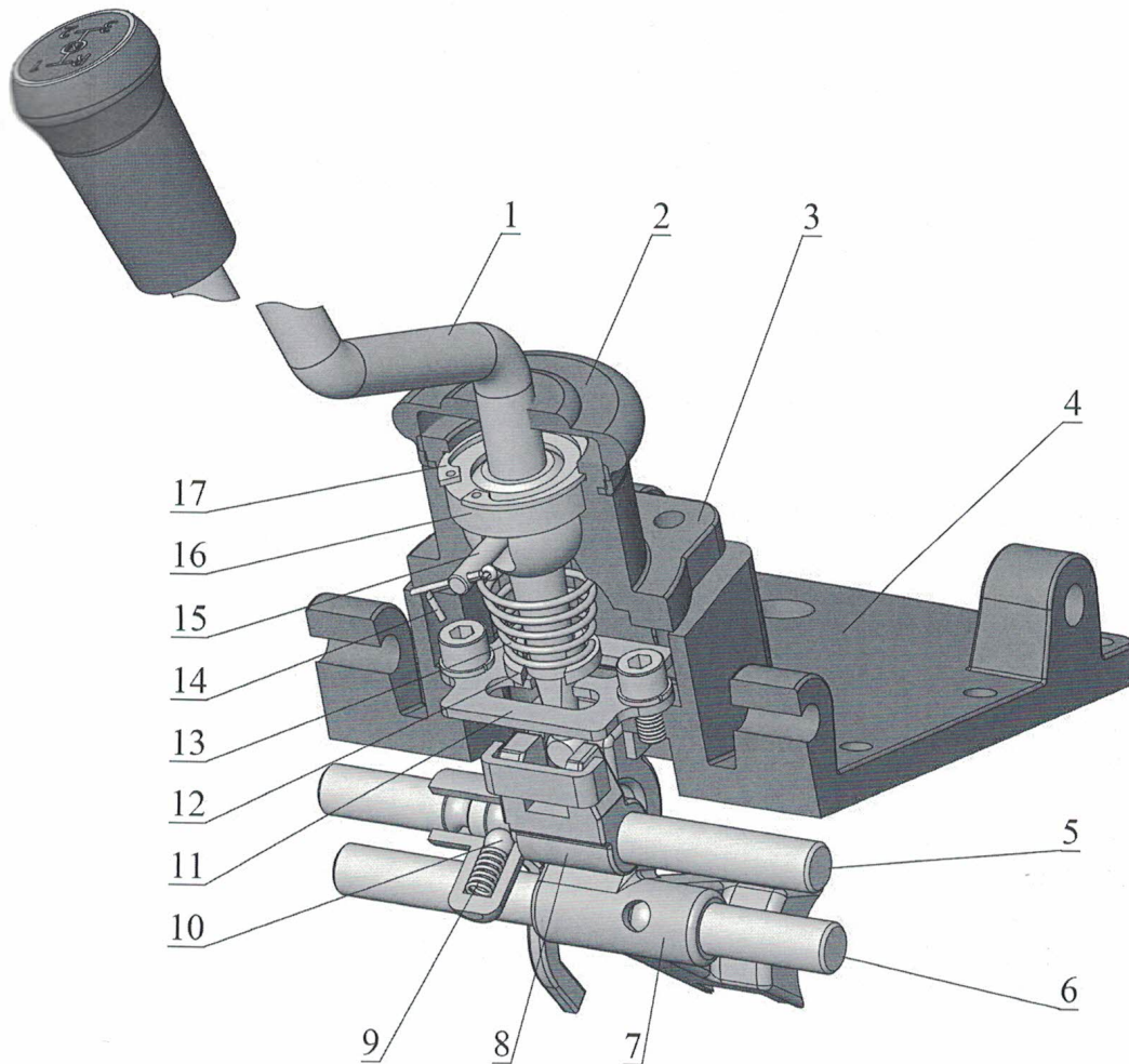
Рис. 8. Устройство механизма переключения передач 1, 2, 3, R
