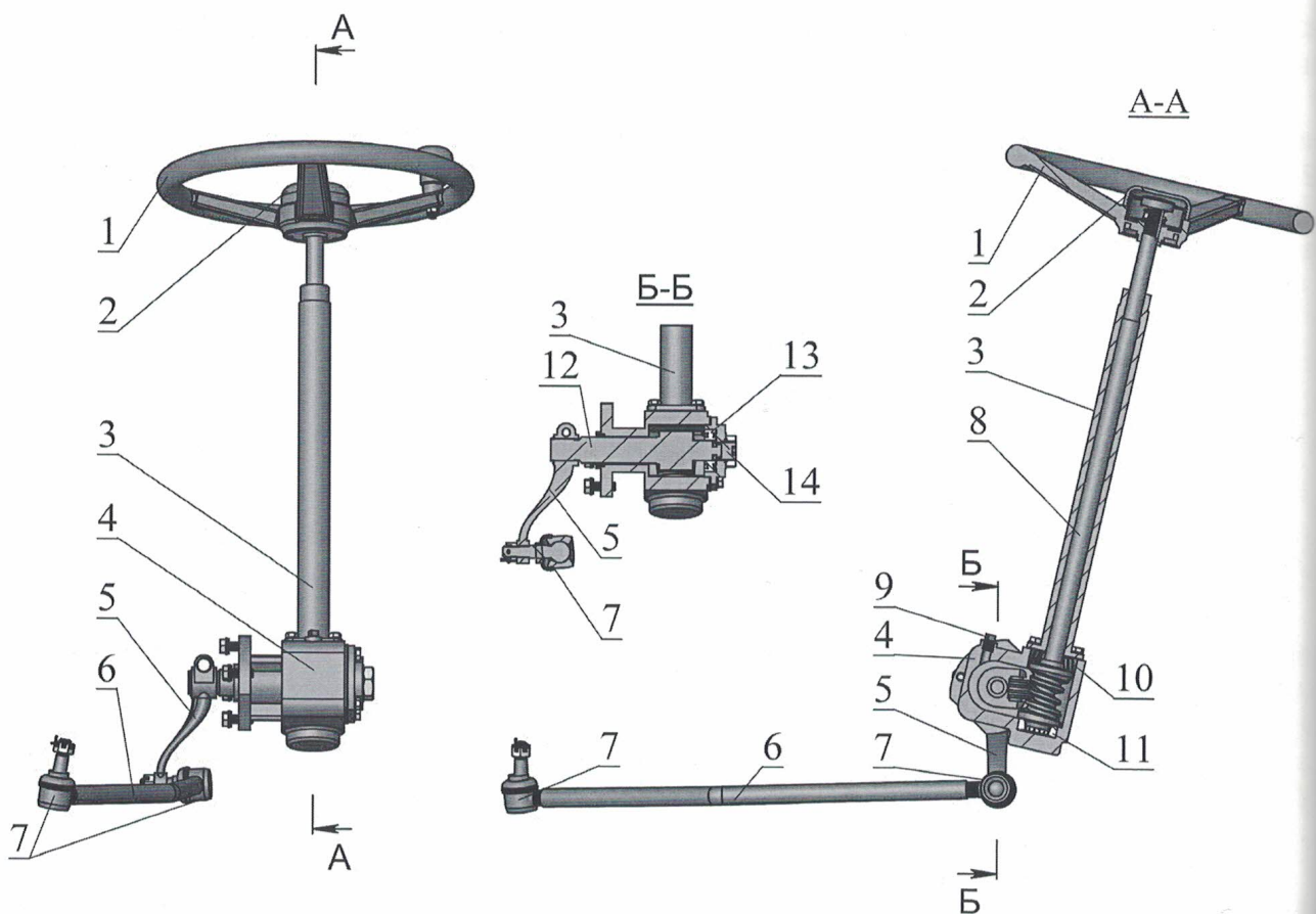
Рис. 19. Рулевой механизм
