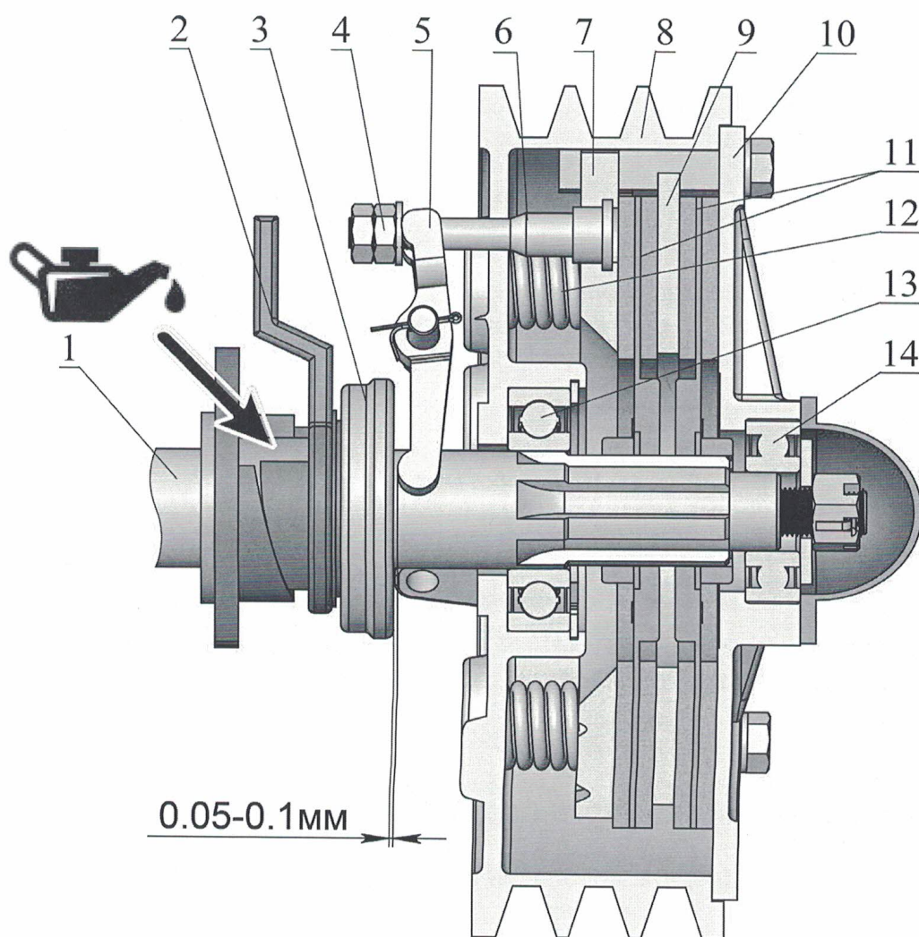
Рис. 10. Устройство муфты сцепления
