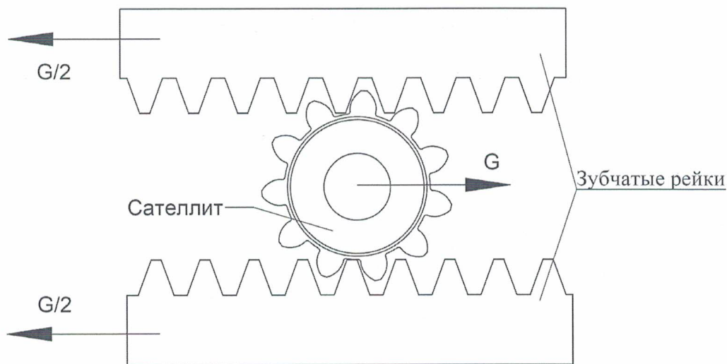
Рис. 6. Схема работы дифференциала
