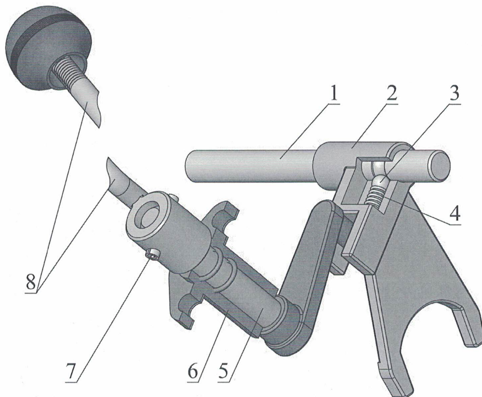
Рис. 9. Устройство механизма переключения повышенных/пониженных передач
