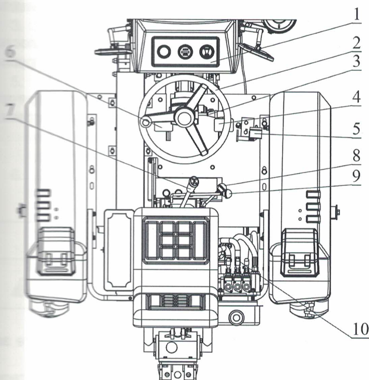
Рис. 2. Органы управления трактором
