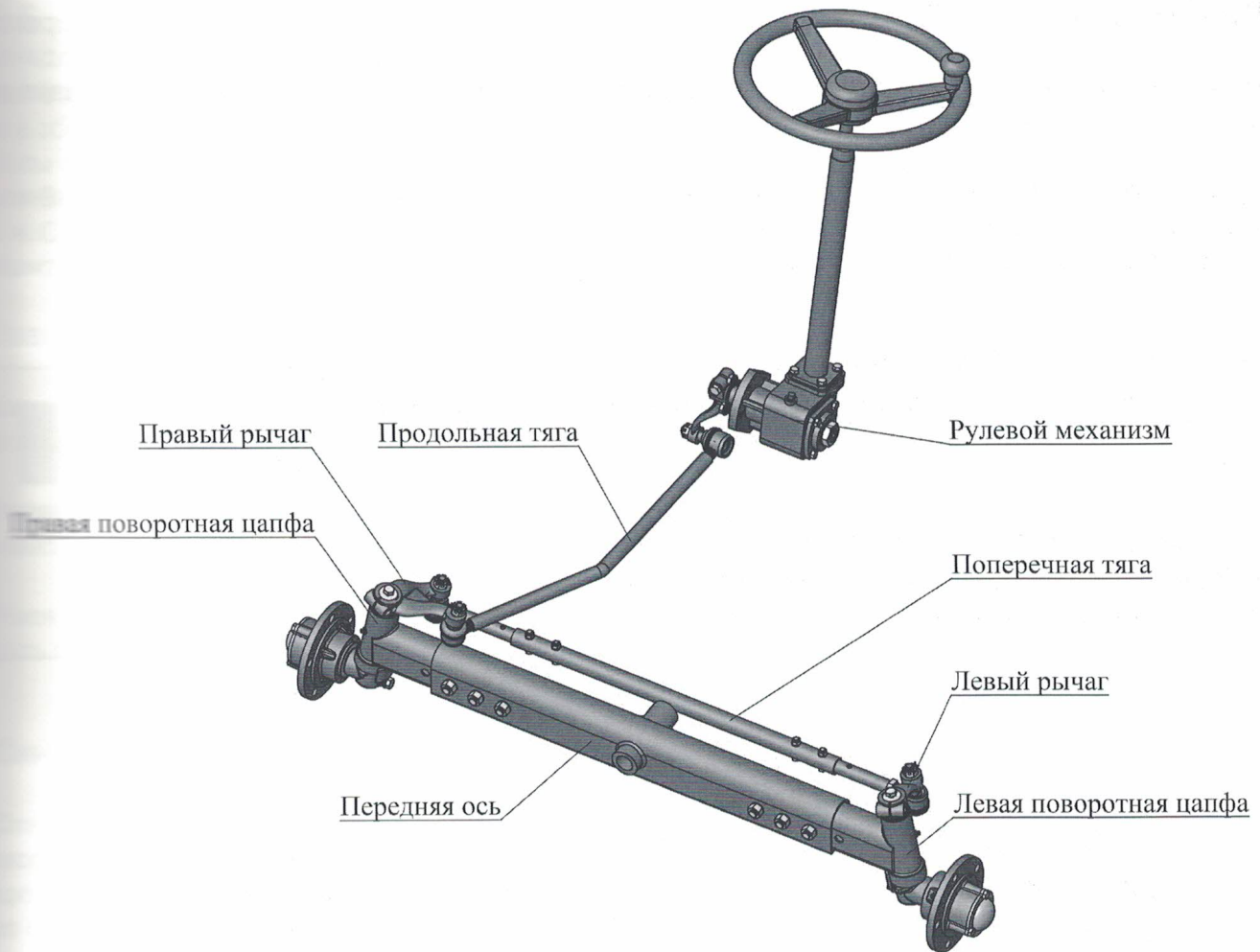
Рис. 20. Рулевой привод
