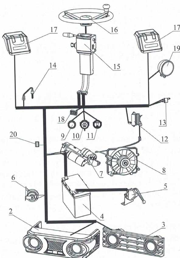
Рис. 23. Схема электрооборудования тракторов ФАЙТЕР
