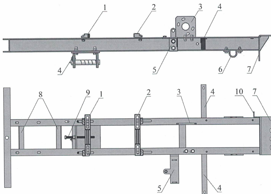
Рис. 13. Рама трактора
