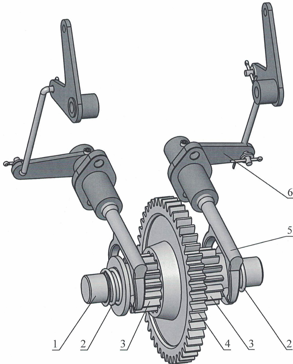
Рис. 4. Устройство механизма блокировки полуосей.
