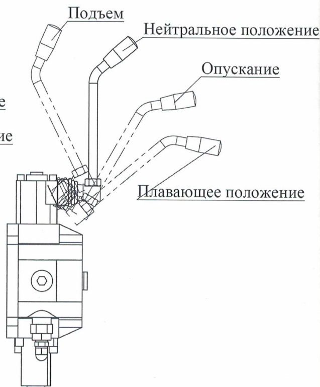
Рис. 24. Схема переключения режимов гидрораспределителей
