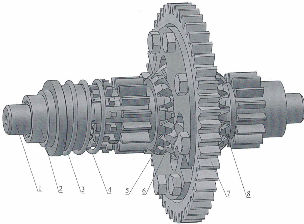
Рис. 5. Устройство дифференциала
