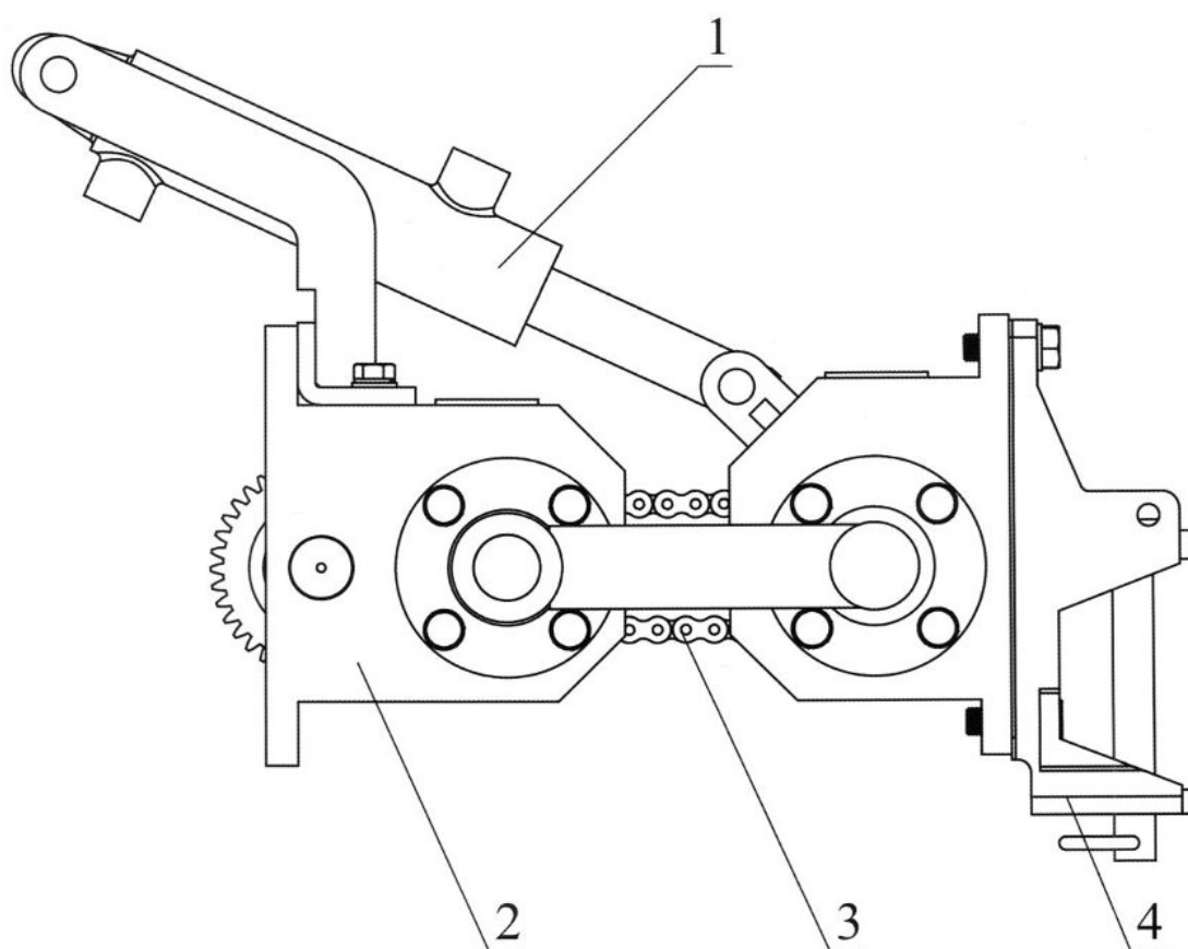
Рис. 25. Редуктор подъемного навесного оборудования
