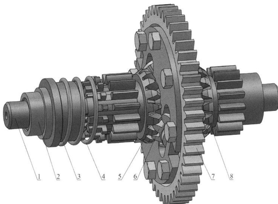
Рис. 5. Устройство дифференциала
