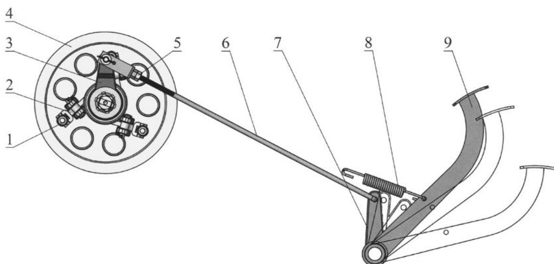
Рис. 11. Настройка муфты сцепления
