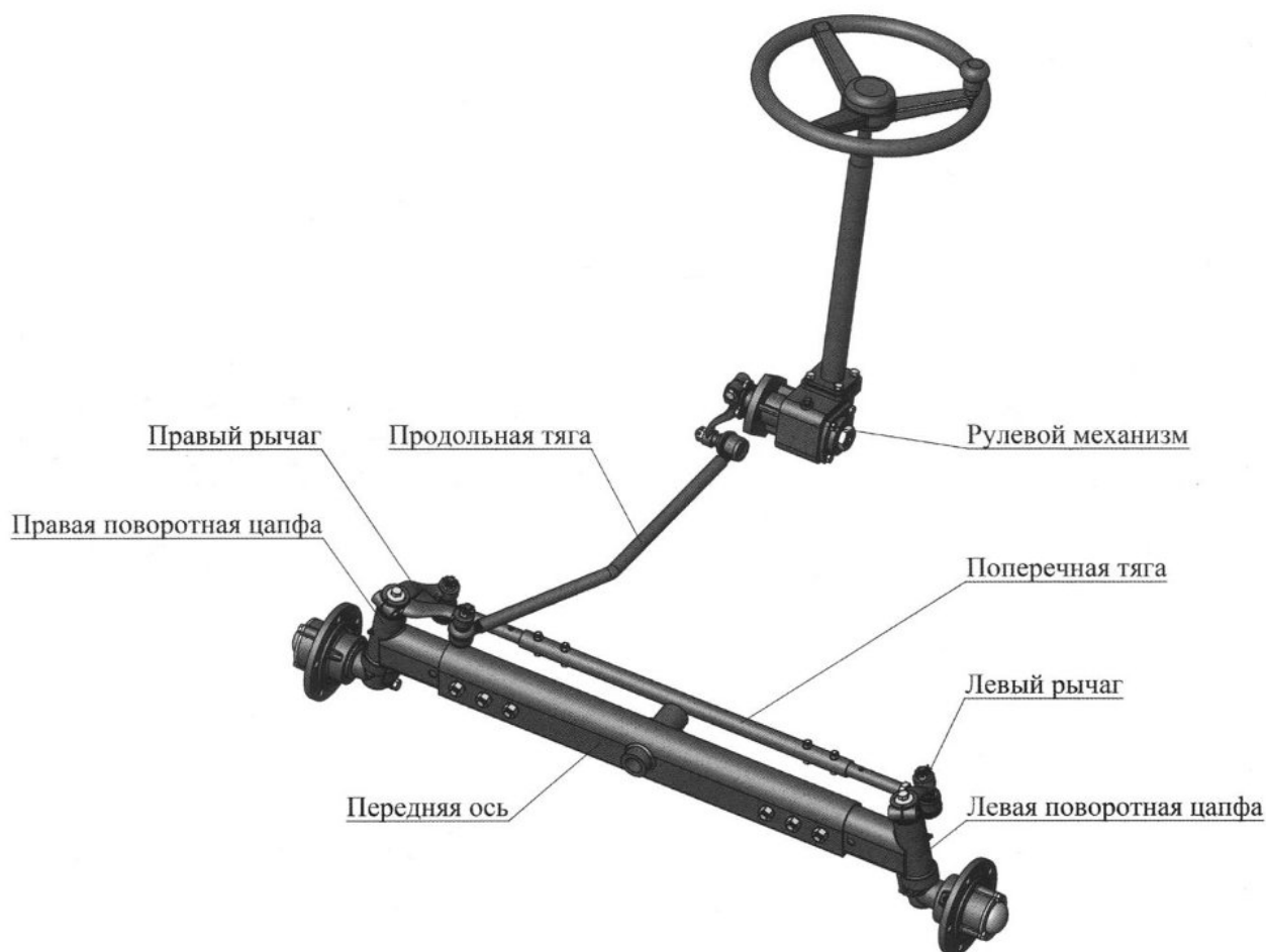
Рис. 20. Рулевой привод
