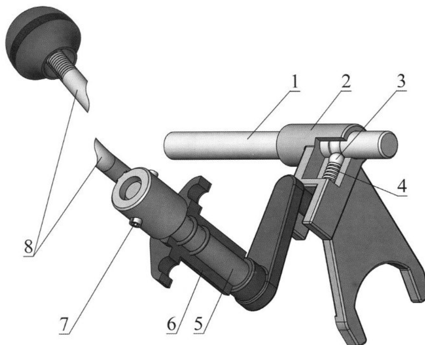
Рис. 9. Устройство механизма переключения повышенных/пониженных передач
