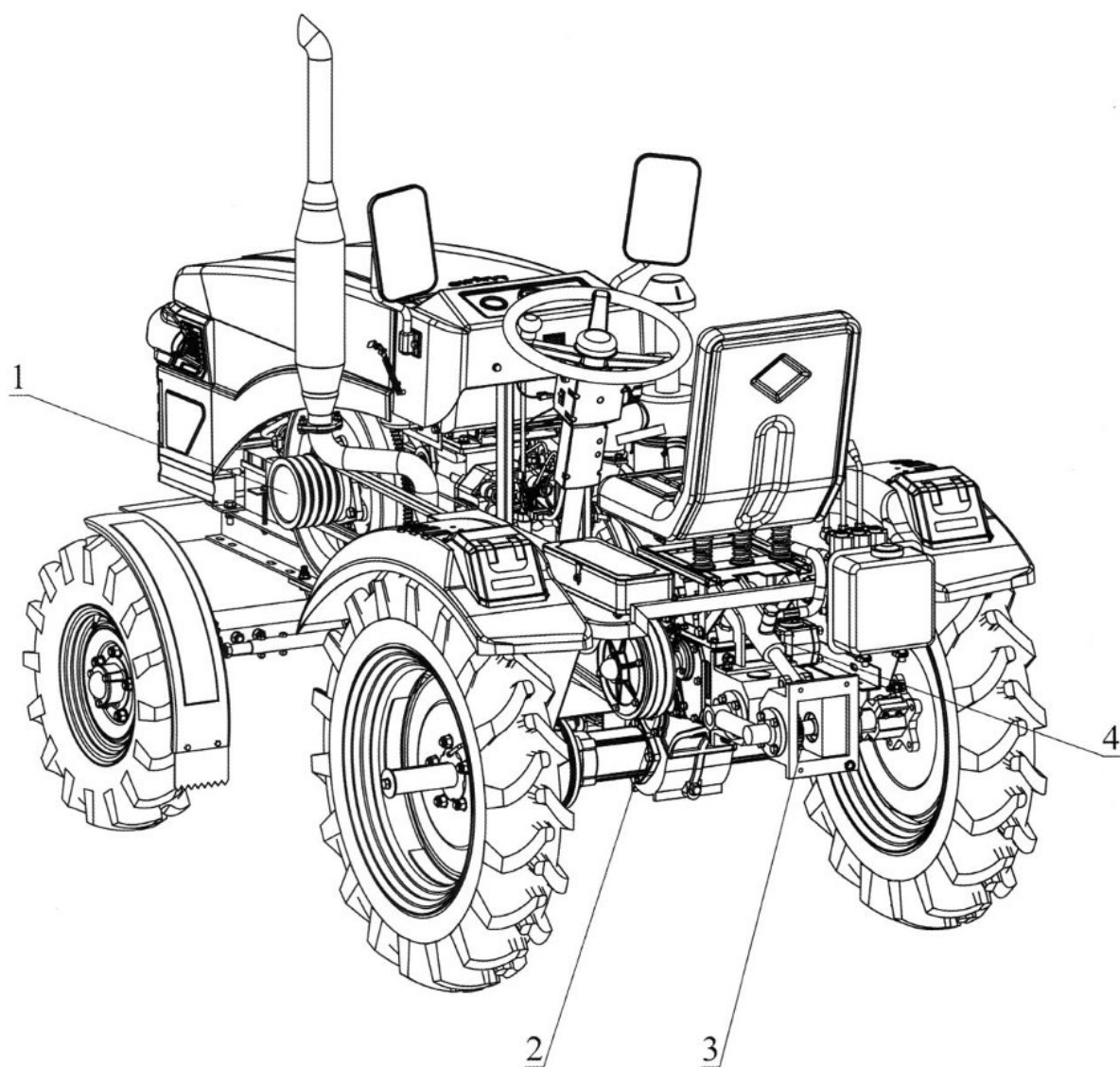
Рис. 22. Расположение валов отбора мощности
