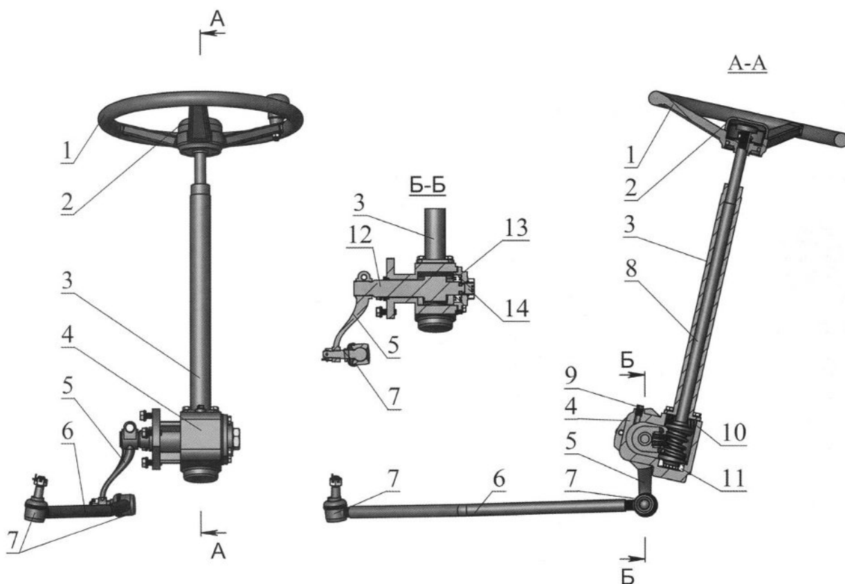
Рис. 19. Рулевой механизм
