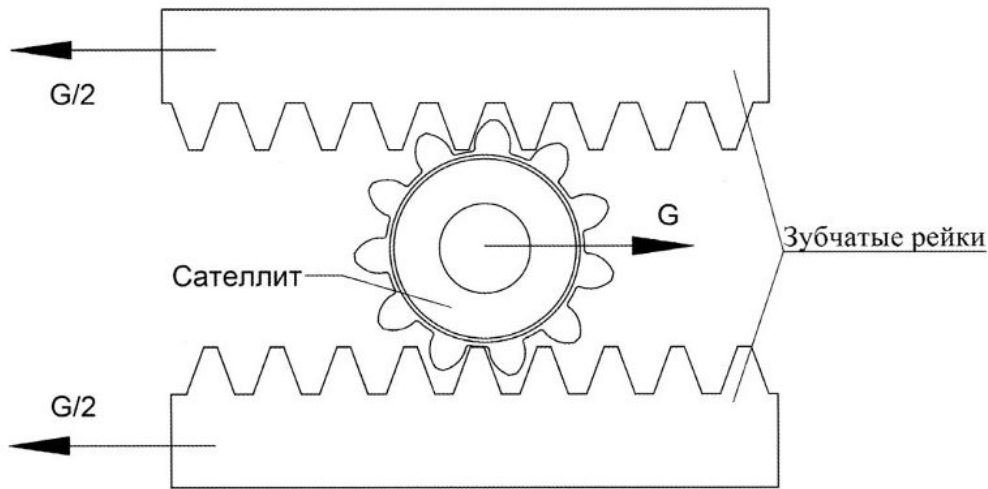
Рис. 6. Схема работы дифференциала
