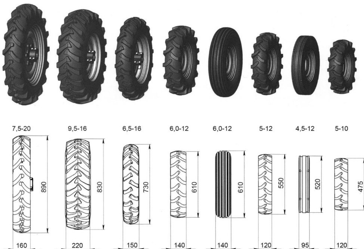
Рис. 18. Размеры колес
