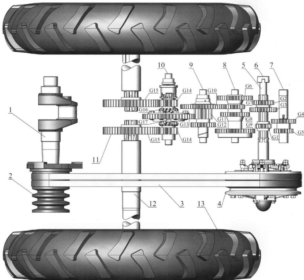
Рис. 3. Схема трансмиссии трактора
