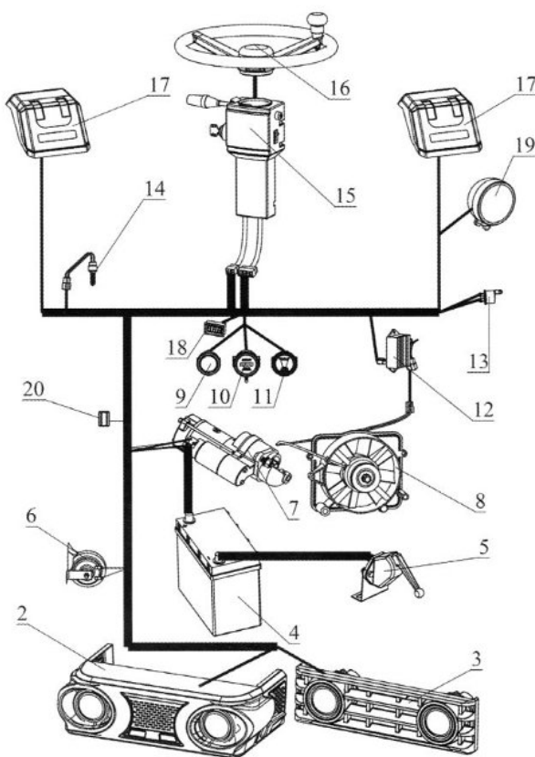
Рис. 23. Схема электрооборудования тракторов TZR
