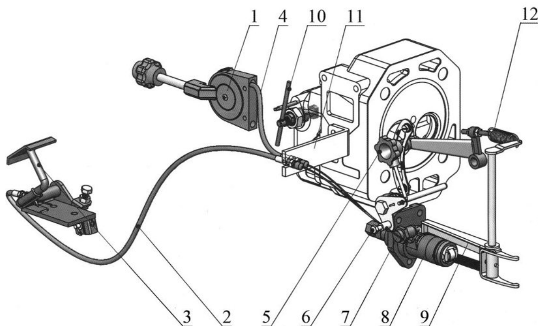
Рис. 21. Органы управления двигателем
