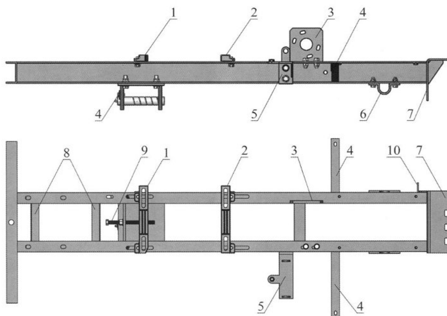
Рис. 13. Рама трактора
