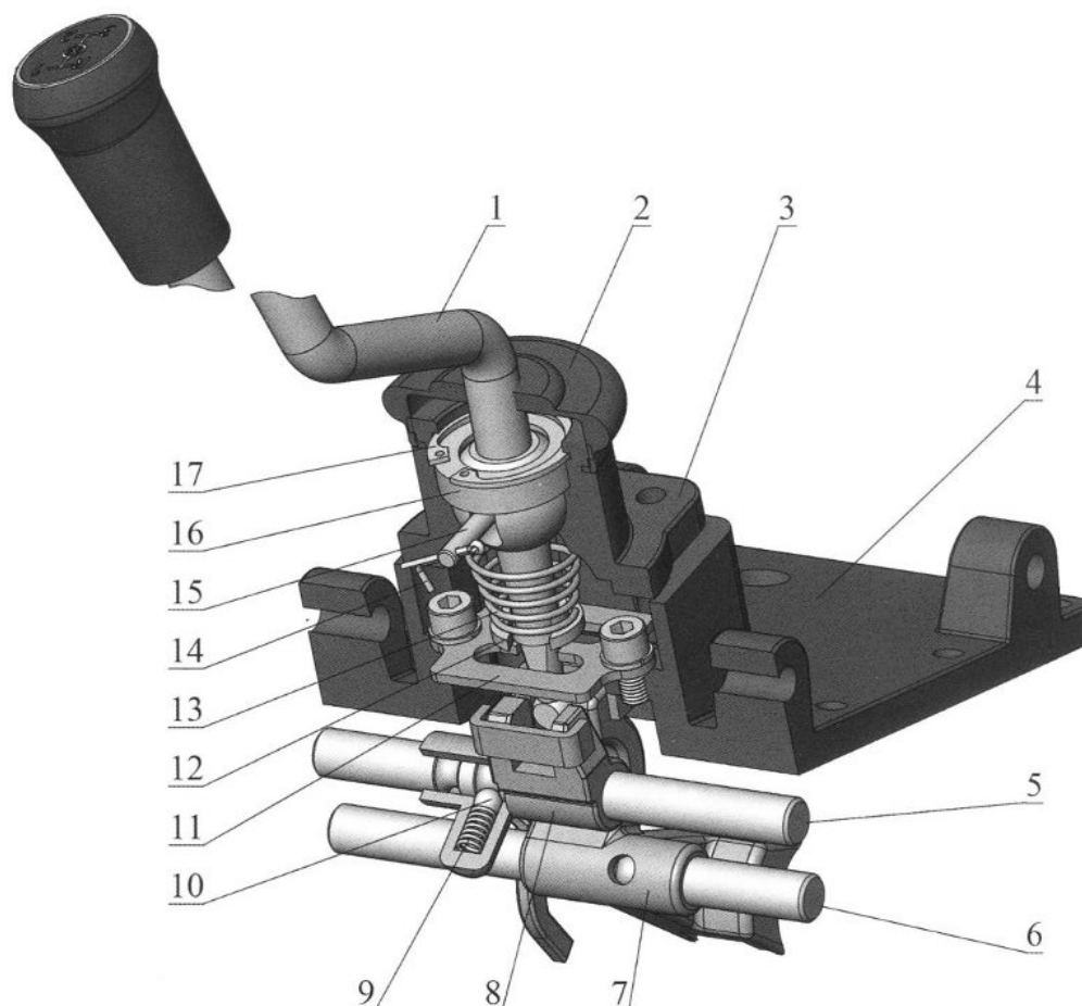
Рис. 8. Устройство механизма переключения передач 1, 2, 3, R
